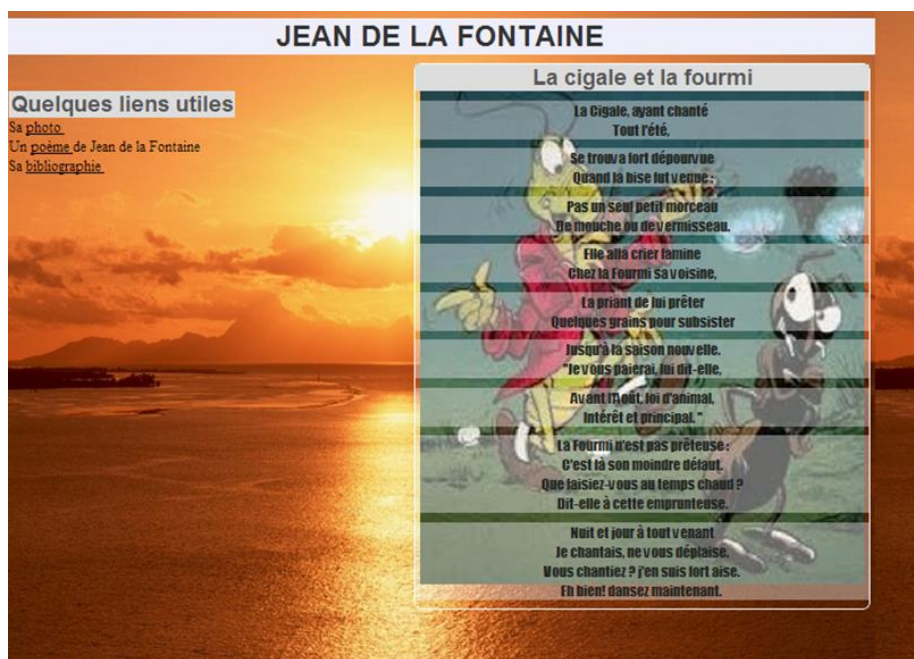
HTML + CSS
